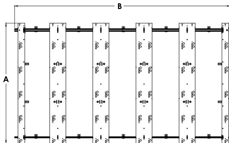
VORDERANSICHT
