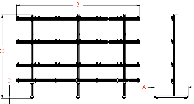
VORDERANSICHT
