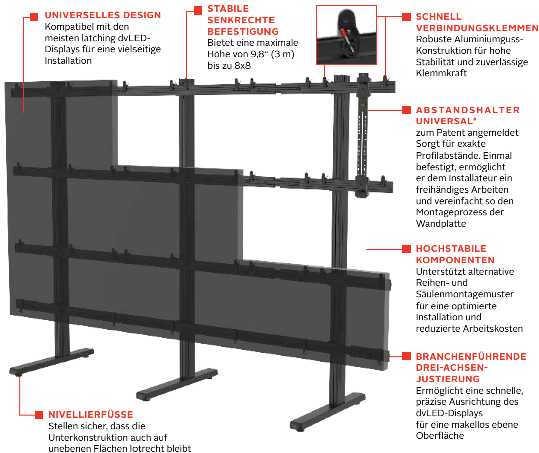
ABBILDUNG ZEIGT LEDFSS-6X6
