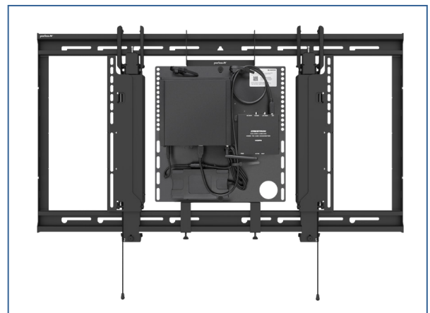
ACC-STSCF1 mit der ultradünnen Wandhalterung Universal mit Scherenmechanismus der SmartMount®-Reihe (STS680) und Creston® Flex 260/200 UC-Montagehalterung
