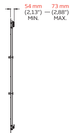
VUE LATÉRALE
