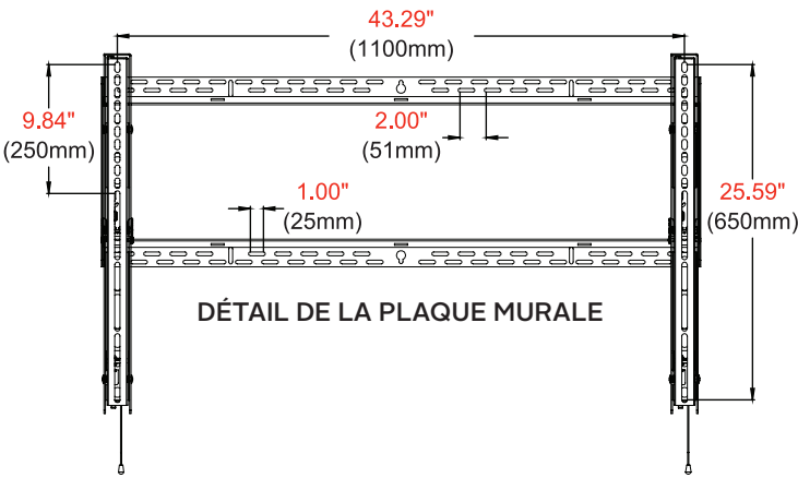
DÉTAIL DE LA PLAQUE MURALE
