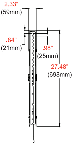
DÉTAIL PLAQUE DE RACCORD
