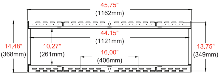
DÉTAIL DE LA PLAQUE MURALE
